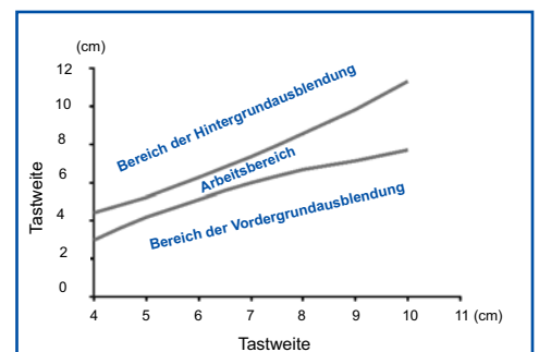
Hysteresis mit EASYtouch™ Einstellung
